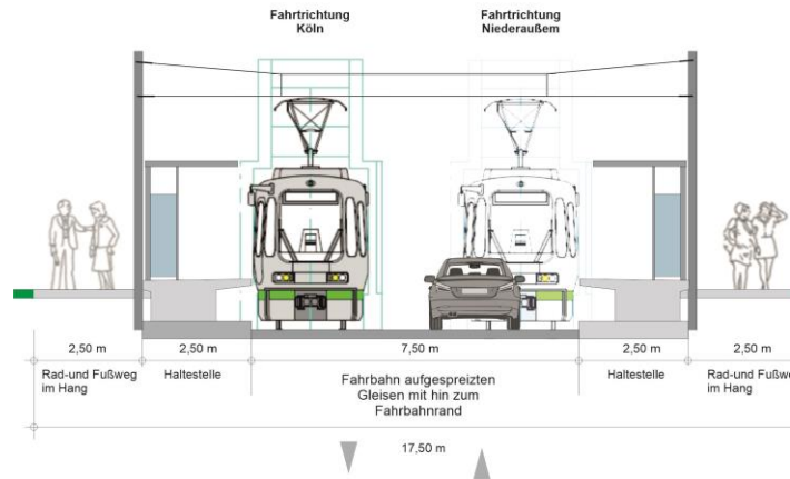
Querschnitt in Oberaußem mit Haltestelle
