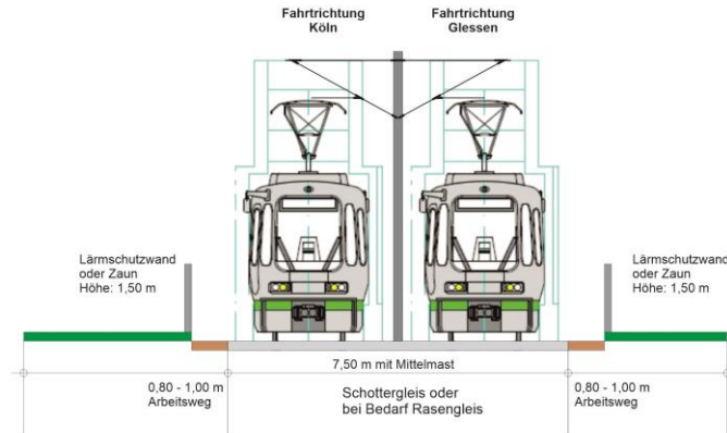
Querschnitt auf freier Strecke (Regelquerschnitt)
