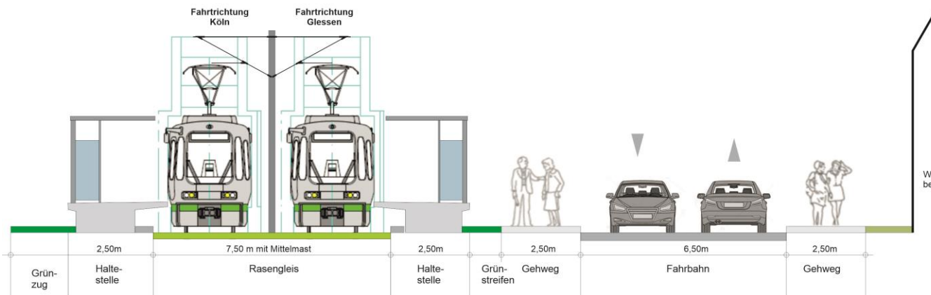
Querschnitt Helmholtzstraße in Brauweiler mit Seitenbahnsteigen
